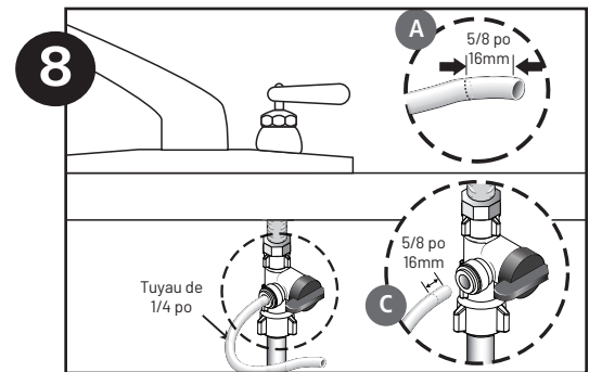
Schéma de raccordement
