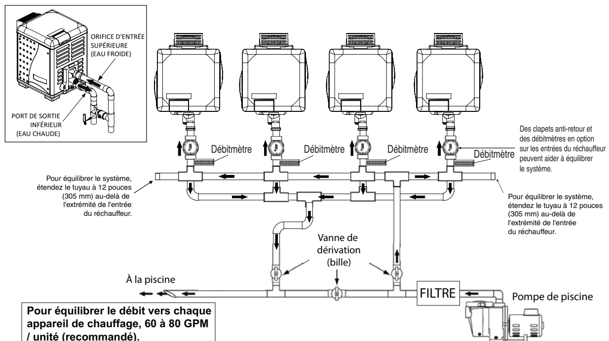
Figure 2. Schéma de plomberie hydraulique des quatre réchauffeurs 125 MasterTemp
