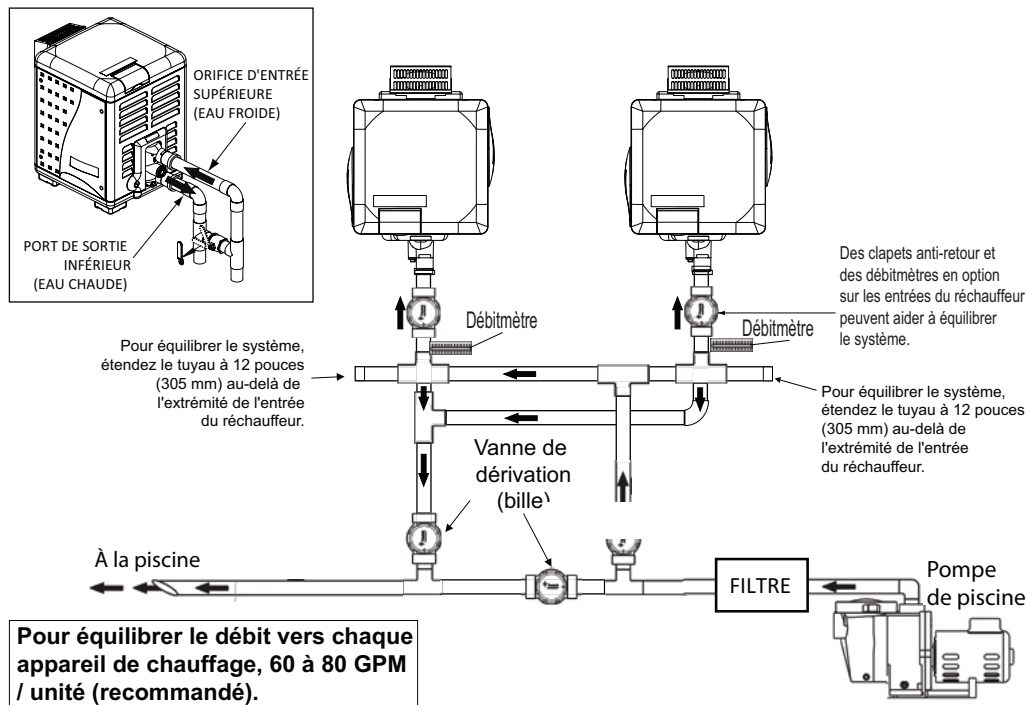
Figure 1. Schéma de plomberie hydraulique des deux réchauffeurs 125 MasterTemp
