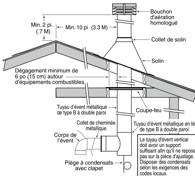
Figure 18. – L'installation de tuyau de conduit en métallique typique - Canada. (Verticale - la Pression Négative)
