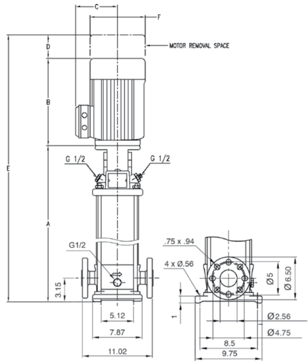
ANSI 250# Flanges
