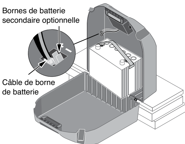
Figure 5 : l'entrée de la batterie se trouve dans le boîtier de la batterie. Soutenir le boîtier lors de son ouverture. Le support doit avoir une épaisseur d'au moins 10,2 cm (4 po).'
