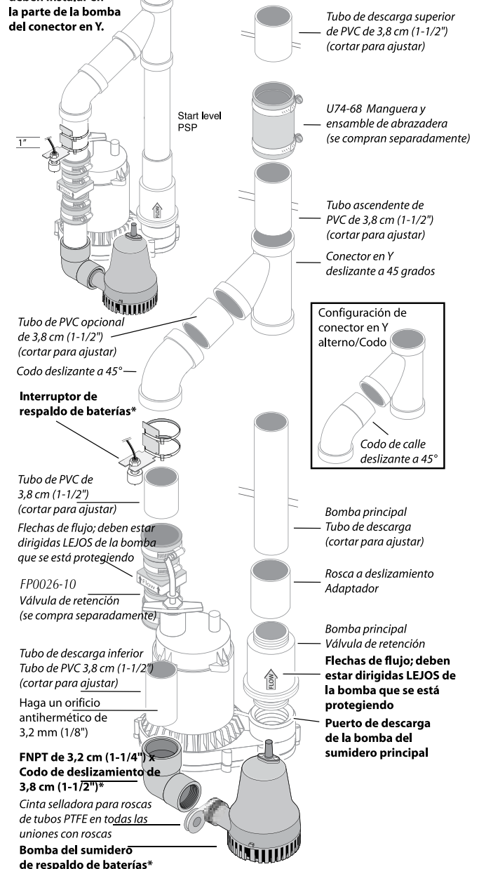
Figura 3: Instalación típica con tubos de descarga comunes.
