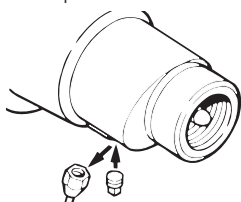
Figura 3 - Tape el orificio de AVC (control del volumen de aire) cuando instale el tanque precargado en bombas ya existentes. Las nuevas bombas vienen con el tapón instalado.
