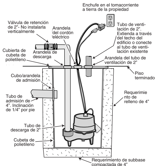
Figura 1 – Instalación típica
