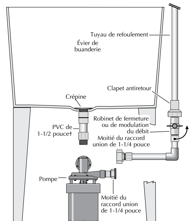
Figure 3 : Dépose de la pompe
