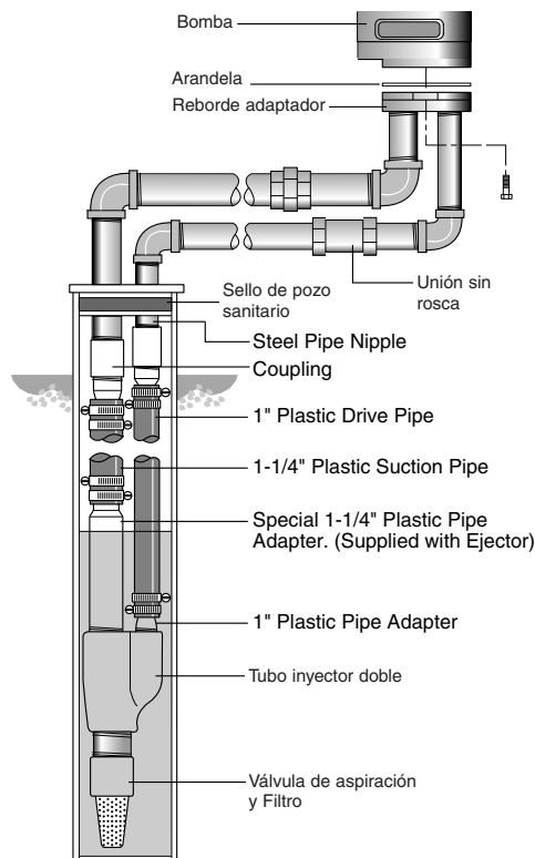
Figura 4 – Instalación desplazada
