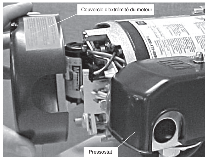
Figure 4 – Dépose du couvercle d'extrémité du moteur
