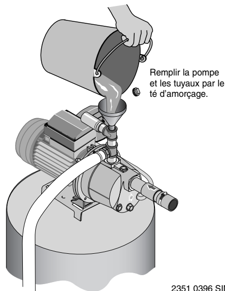
Figure 8 : Amorçage de la pompe
