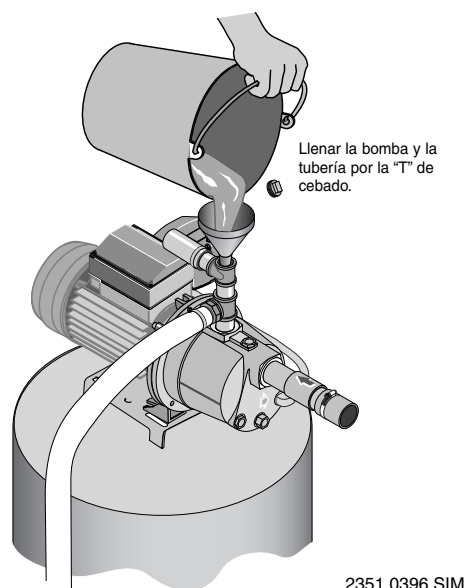
Figura 8: Llenado de la Bomba
