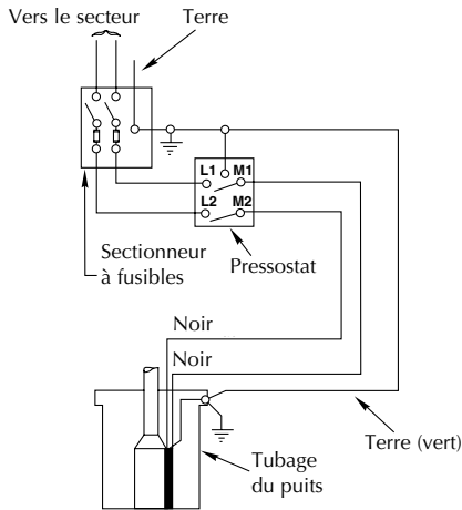
FIGURE 1B - Courant monophasé, mises à la terre à 2 fils. Les pompes à 2 fils comportent deux fils branchés entre le courant électrique (noir) et un fil de mise à la masse (vert). La boîte de commande n'est pas nécessaire. C'est l'information correcte seulement pour le raccordement des moteurs à 2 fils de 115 et de 230 volts.
