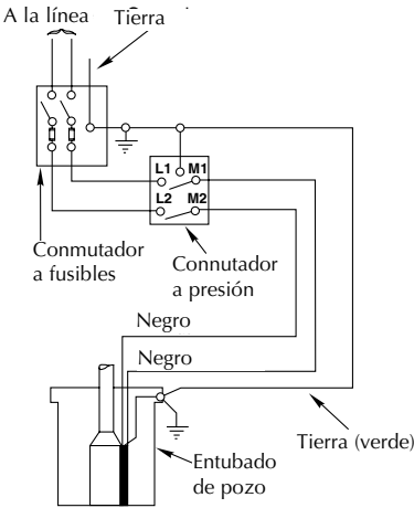
Figura 1B - Las bombas bifilares con conexiones monofásicas y bifilares tienen dos hilos de suministro de corriente (negro) y un hilo de puesta a tierra (verde). No se requiere una caja de control. Esta es la información correcta sólo para las conexiones de motores bifilares de 115 y 230 voltios.
