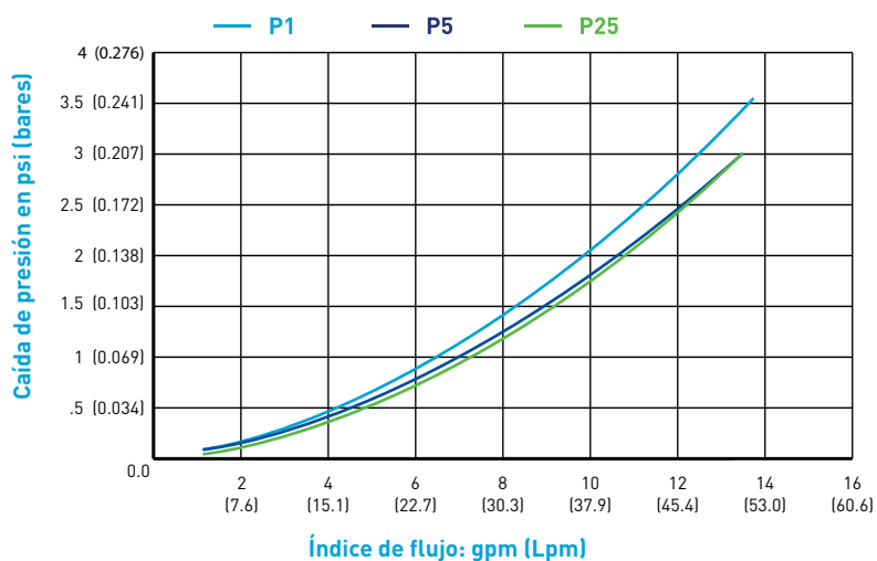
Serie P: Caída de presión y caudal
