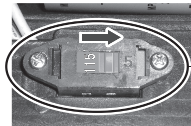
Figure 12B : La tension est réglée à 115 V (comme ci-dessus) en usine. Pour changer la tension, glisser le commutateur de façon à ce que le chiffre « 230 » soit visible (comme ci-dessous).
