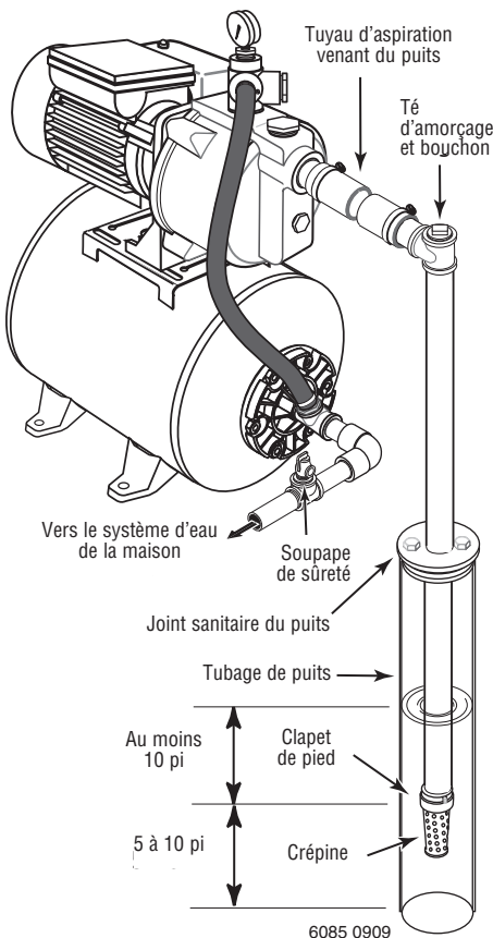
Figure 2 : Installation dans un puits à tubage
