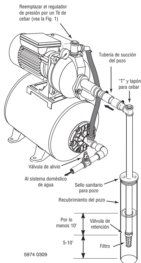
Figura 7 : Instalación de Pozo Recubierto
