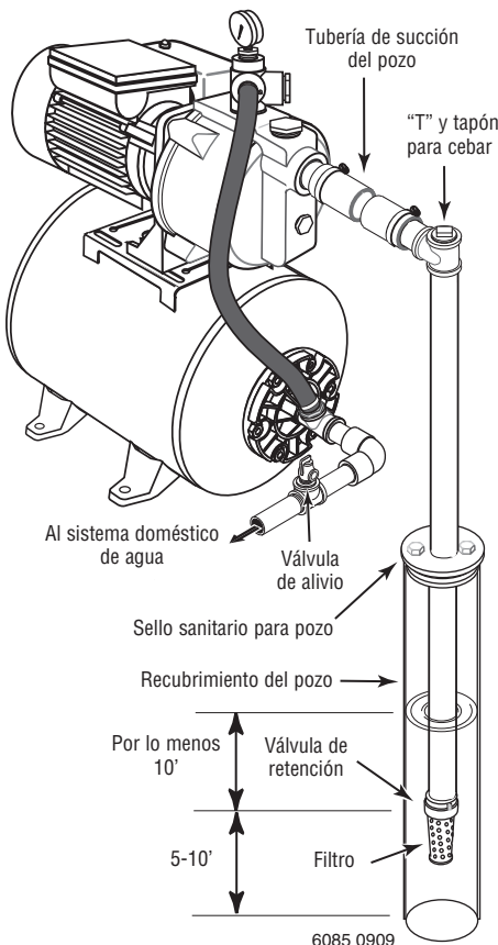
Figura 2: Instalación de pozo recubierto
